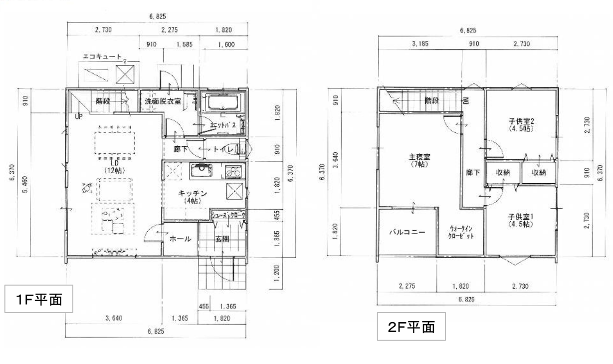
【間取り図】
